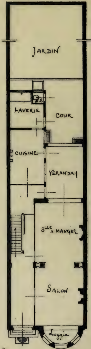
REZ-DE-CHAUSSÉE
